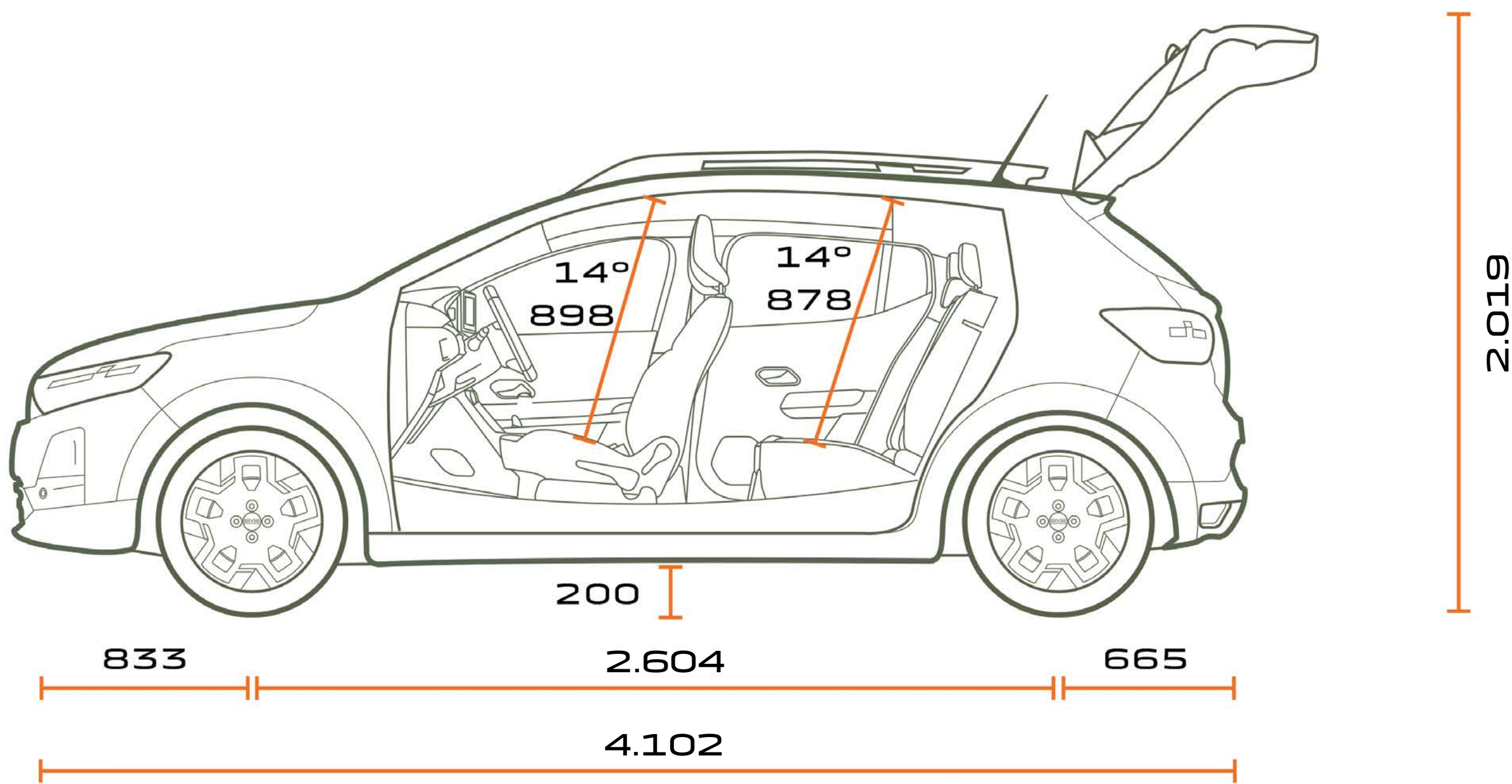
VEDERE LATERALĂ
