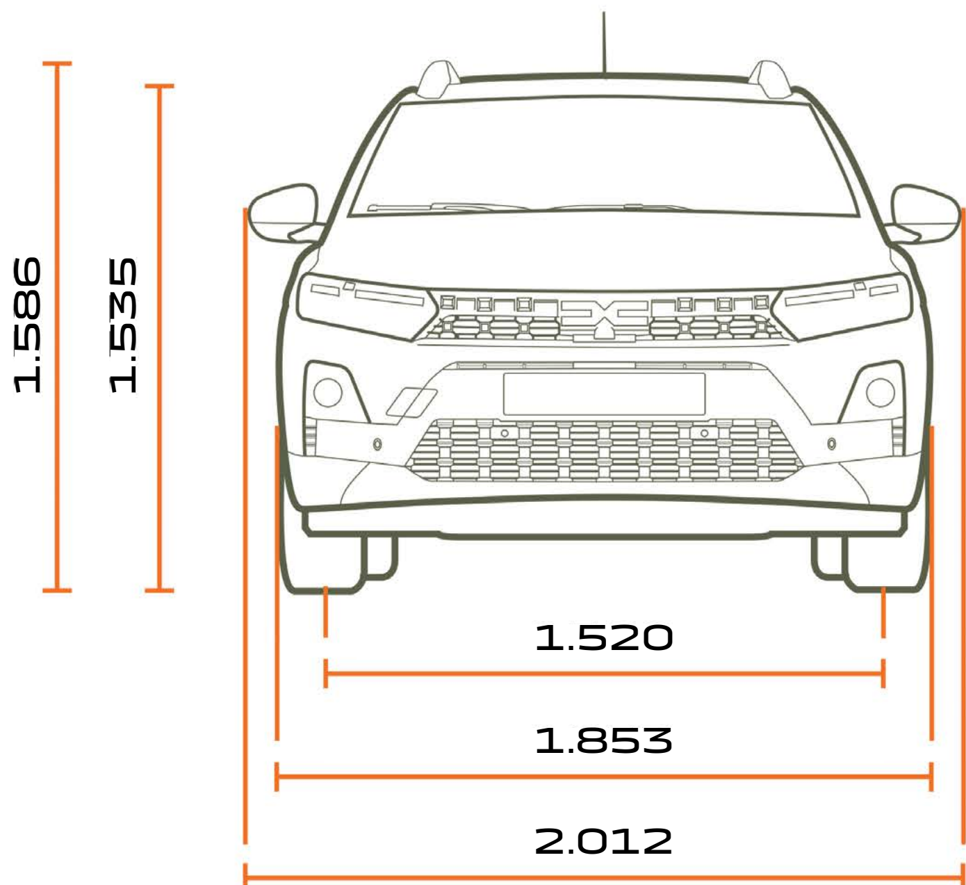
VEDERE FRONTALĂ
