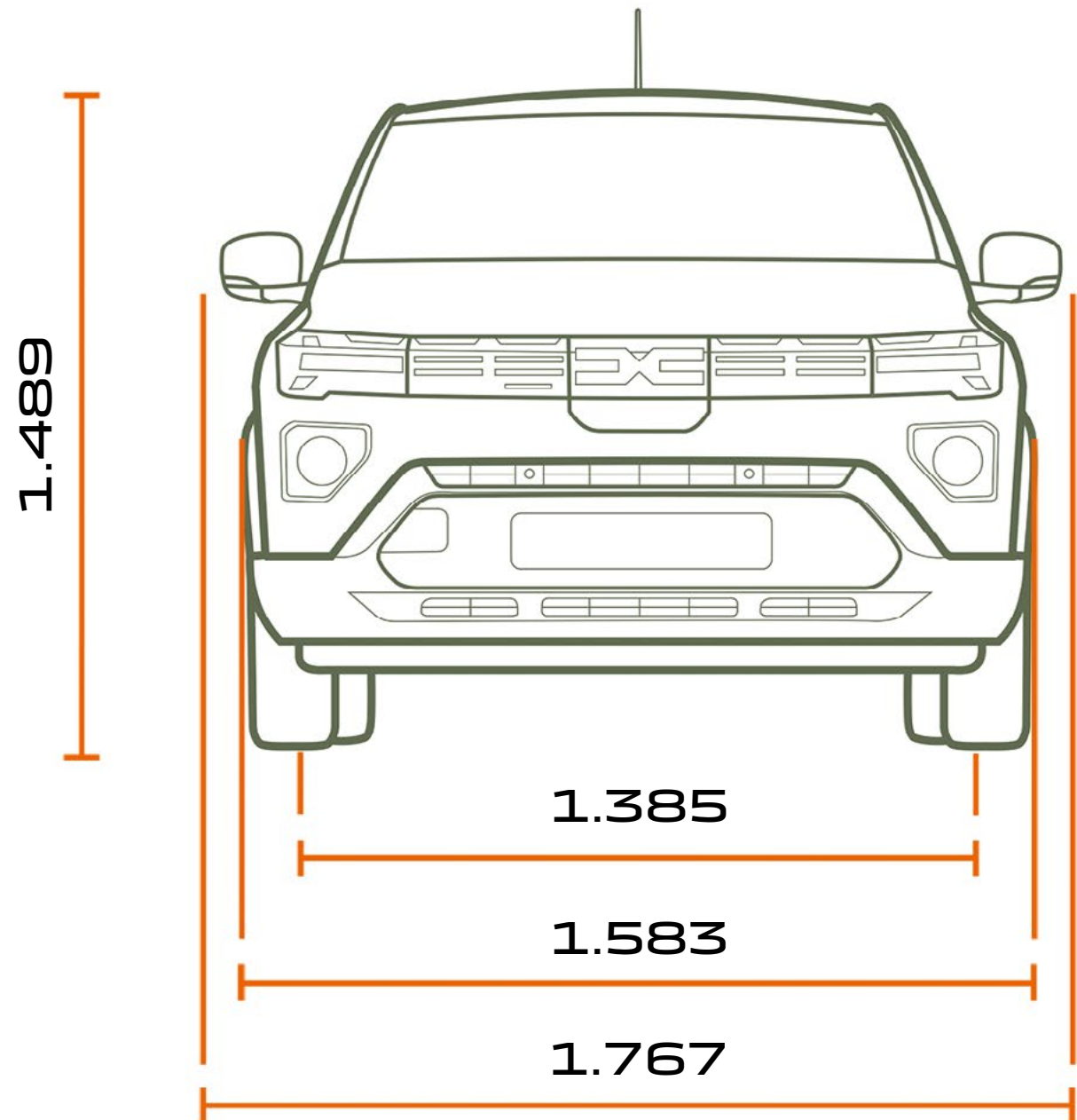
VEDERE FRONTALĂ
