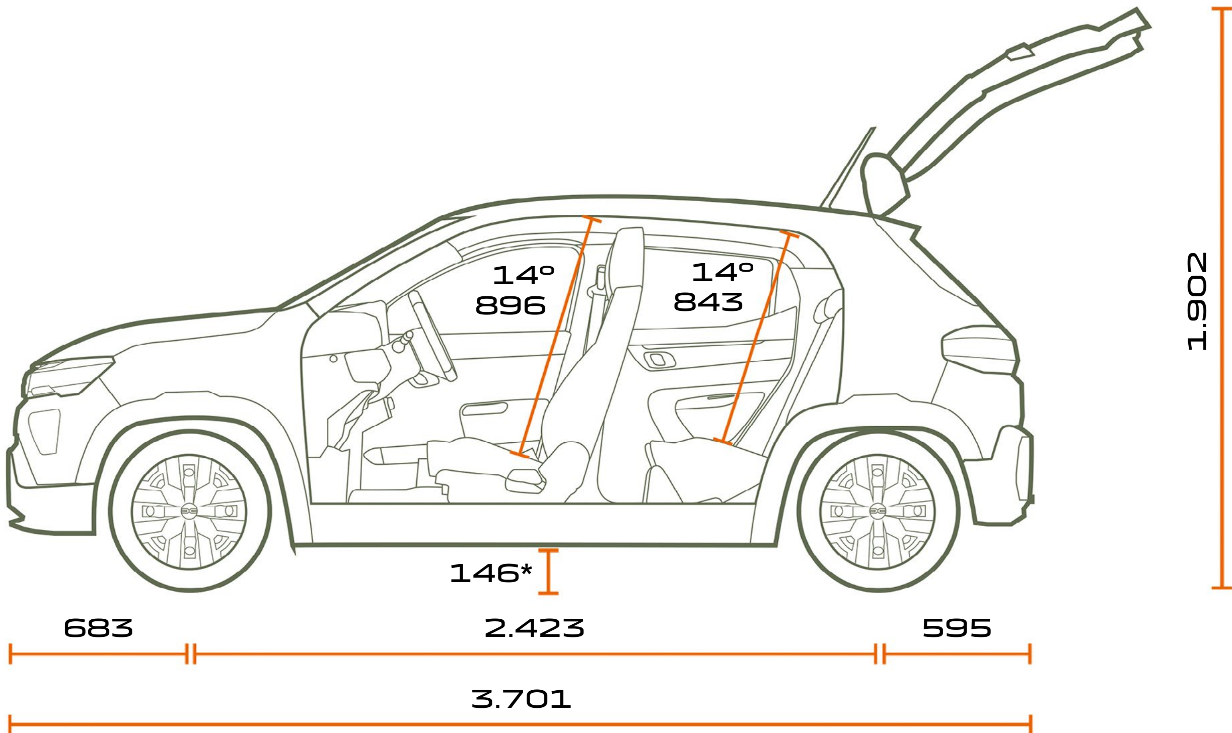
VEDERE LATERALĂ
