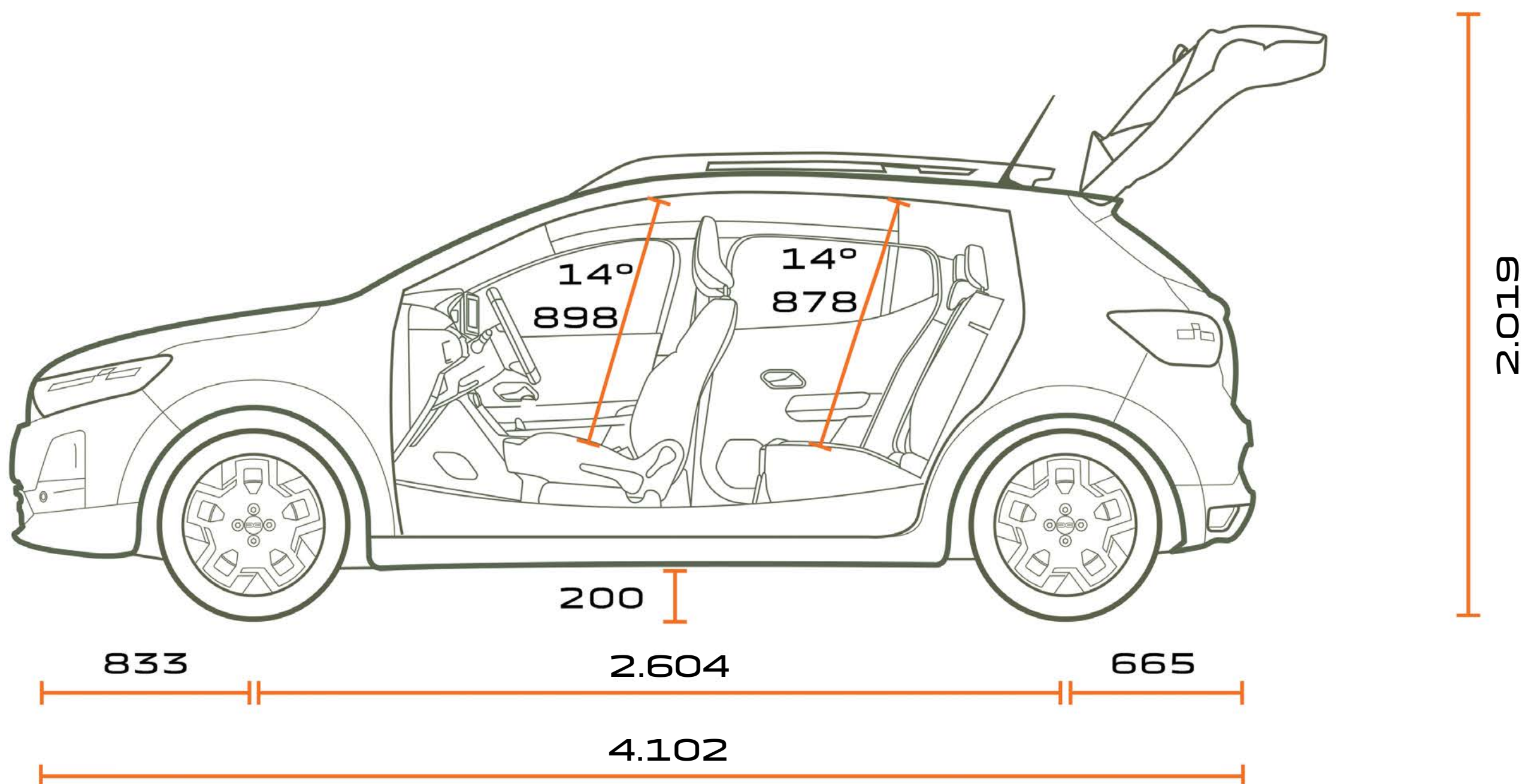
VEDERE LATERALĂ
